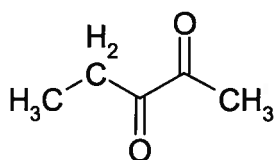
2,3-Pentanedione C 5 H 8 O 2
